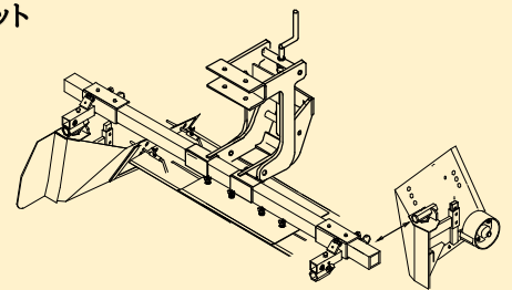
成形部 カチャスポ脱着
