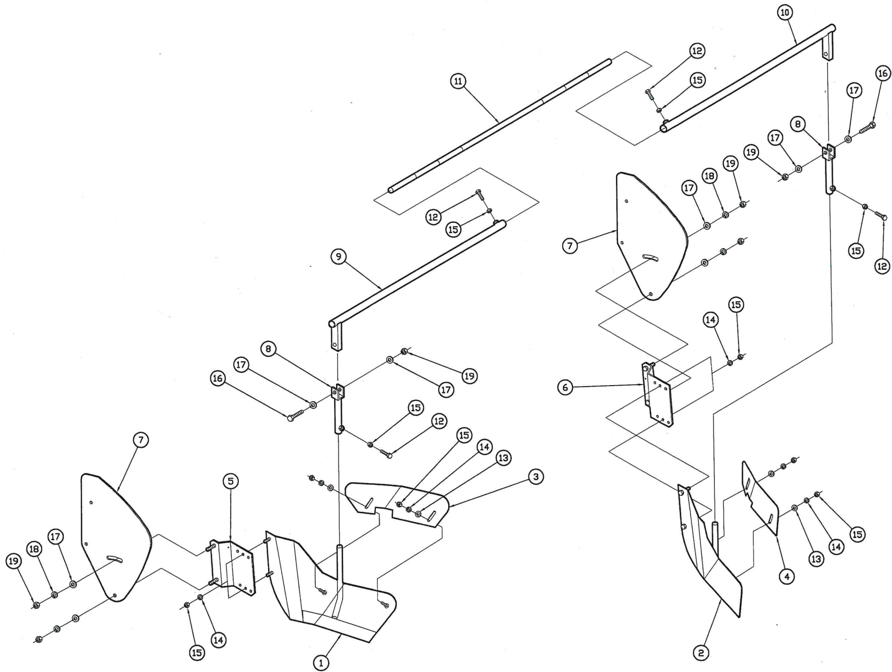
型式 UM3-GX-X 名称 畦盛板3型
